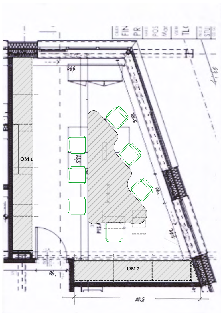
PISARNA 1- DISPOZICIJA OMAR OM1 IN OM2 TER SEJNE MIZE
