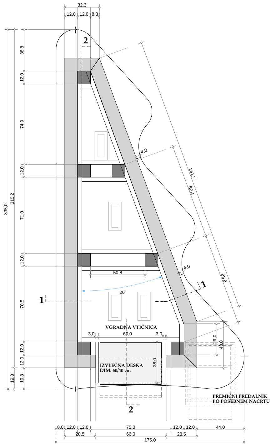
PENT-SEJNA MIZA-PREDLOG PODNOŽJA
