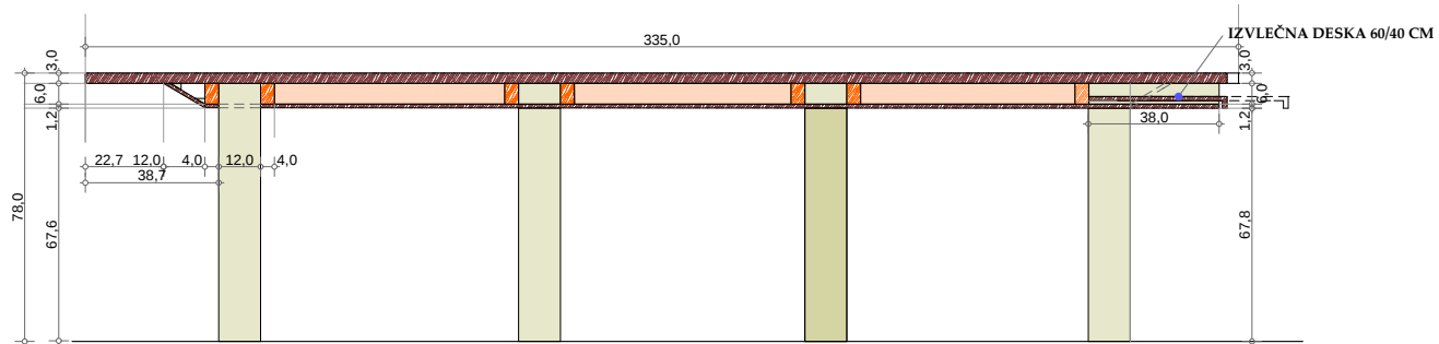
VZDOLŽNI PREREZ MIZE 2-2
