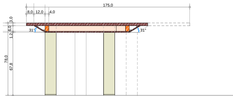
PREČNI PREREZ MIZE 1-1
