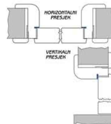
VRATA S IZVUČENIM KRILOM I ZAOBLJENIM DOVRATNIKOM
