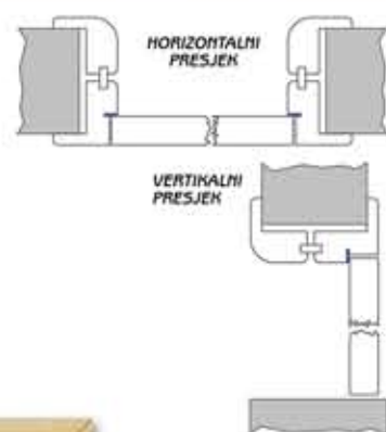
VRATA S DUPLIM DOVRATNIKOM
