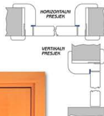
VRATA S UVUČENIM KRILOM I ZAOBLJENIM DOVRATNIKOM
